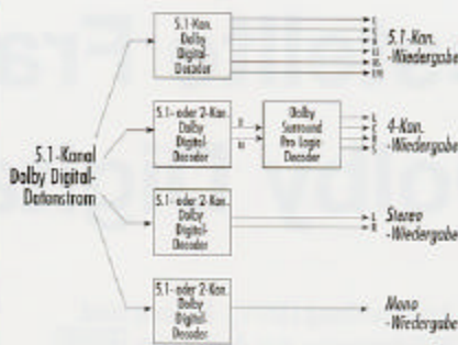
Abbildung 2: Dolby Digital-Decoder passen die Tonsignale automatisch an die jeweiligen Wiedergabe-Bedingungen an.
