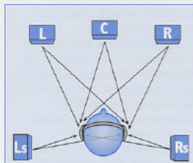
Abbildung 18: Dolby Headphone sorgt für überzeugenden Surround-Sound über konventionelle Stereo-Kopfhörer, indem es den Wiedergabesignalen die besonderen Klangeigenschaften von Lautsprechern in einem Hörraum aufprägt.
